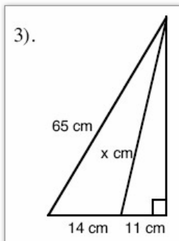
pythag 04
